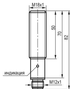
Габаритный чертеж
